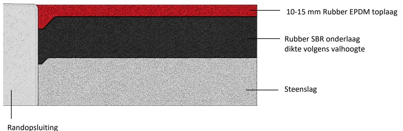
Figuur 2: Onderbouw = steenslag
