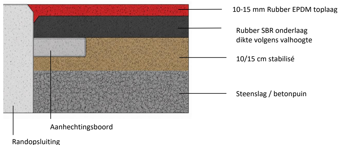
Figuur 1: Onderbouw = stabilisé of chape
